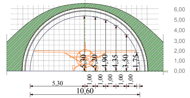
A HANGÁR KERESZTMETSZETE ÉS JELLEMZŐ FŐ MÉRETEI
