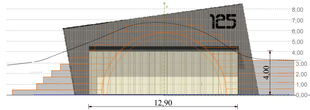
A HANGÁR KERESZTMETSZETE ÉS JELLEMZŐ FŐ MÉRETEI
