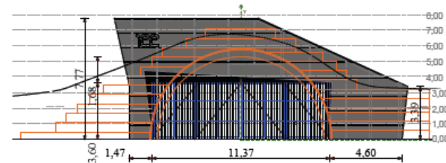
A HANGÁR KERESZTMETSZETE ÉS JELLEMZŐ FŐ MÉRTEI
